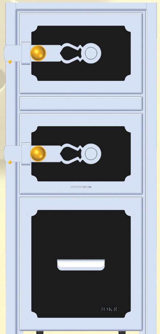
296 - Štít příkládací s uhlákem stavební rozměr š310 x v760 vnější rozměr š350 x v770 x h1535
