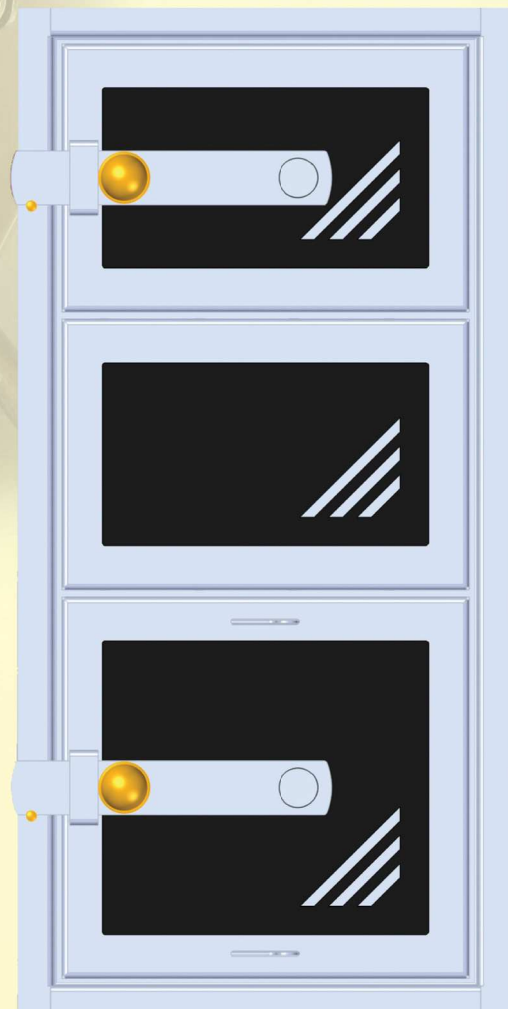
3010 - Štít příkládací burnet stavební rozměr š310 x v680 vnější rozměr š350 x v710
