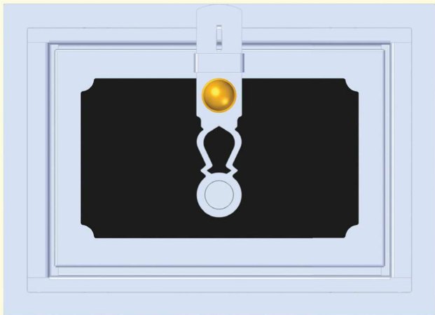
240 - Trouba pečící stavební rozměr š400 x v270 vnější rozměr š457 x v330 x h1515
