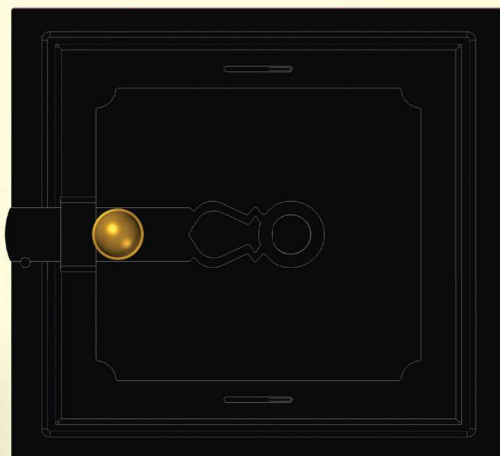
3404 - Dvířka popelníková burnet stavební rozměr š310 x v290 vnější rozměr š350 x v320 x hl55
