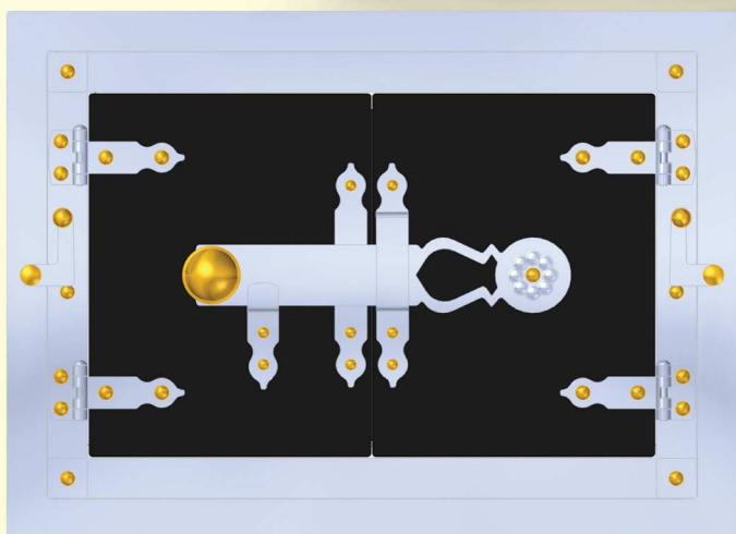
71 - Ohřívárna stavební rozměr š400 x v270 vnější rozměr š457 x v330 x hl510
