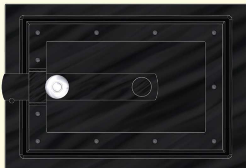
3400 - Dvířka příkladací stavební rozměr š310 x v210 vnější rozměr š350 x v240 x hl55
