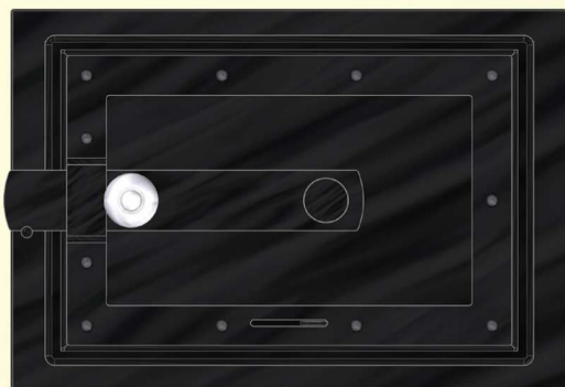
3404 - Dvířka popelníková stavební rozměr š310 x v210 vnější rozměr š350 x v240 x hl55
