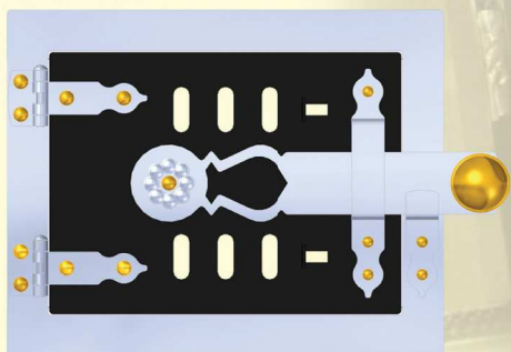
152 - Dvířka popelníková stavební rozměr š210 x v158 vnější rozměr š267 x v212
