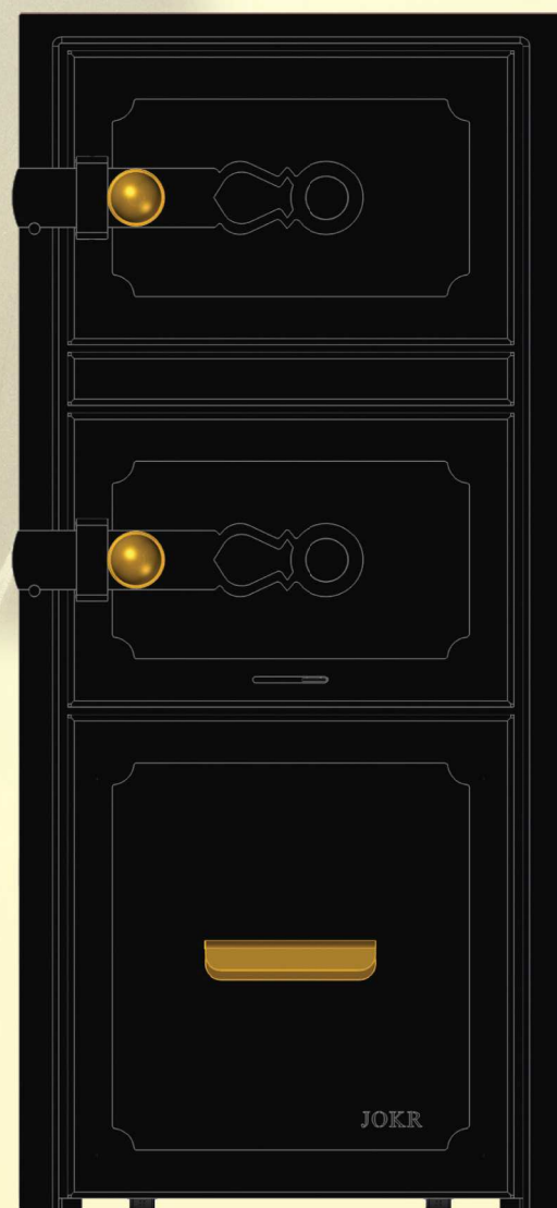
3320 - Štít příkladací s uhlákem stavební rozměr š310 x v760 vnější rozměr š350 x v770 x hl535
