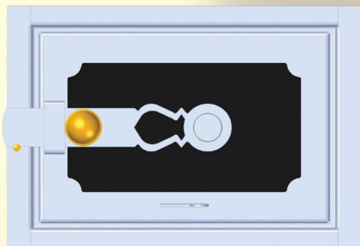
281 - Dvířka popelníková stavební rozměr š310 x v210 vnější rozměr š350 x v240 x h155
